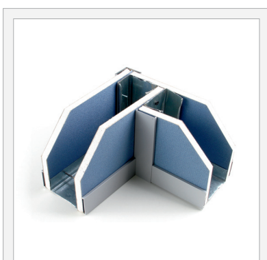
Угловое соединение модулей под углом 90*
