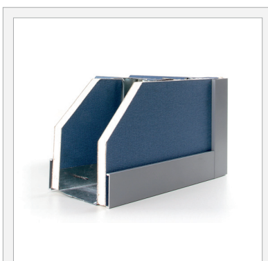
Крепление клипс к каркасному профилю через гипсовинил
