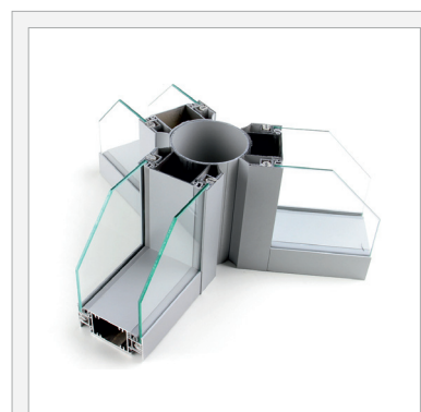
Соединение модулей под произвольным углом
