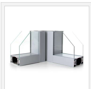
Угловое соединение модулей (внутренний угол)
