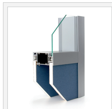
Установка гипсовинила непосредственно в паз профиля
